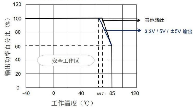
温度降额曲线图（不带散热片）
